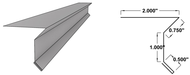
Rake Edge
